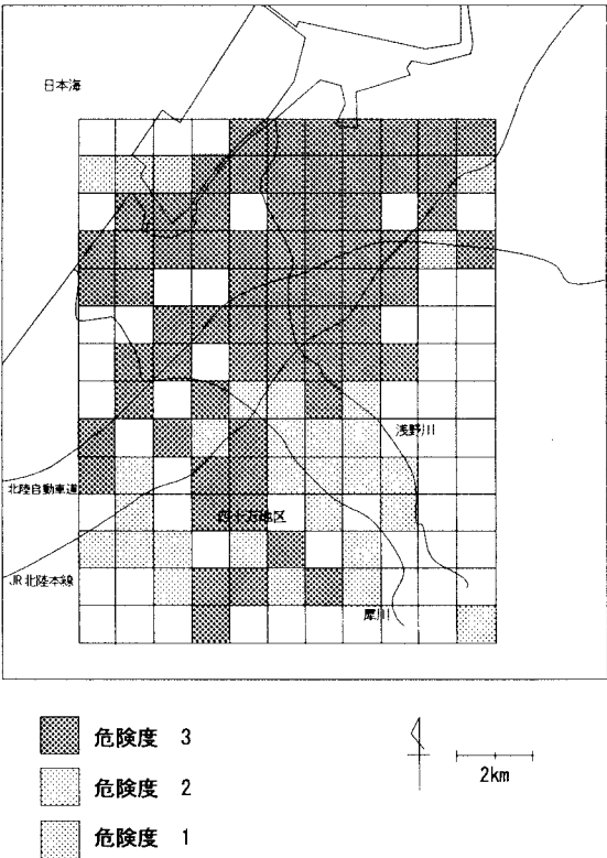
図-3 液状化危険度に基づく地震被害ポテンシャルマップ
