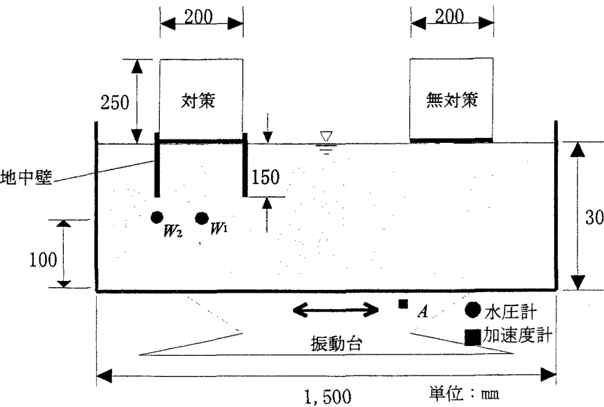
図1 実験概要図
