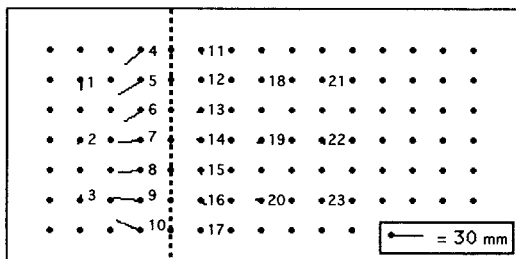
図-4 地表面の水平変位分布
