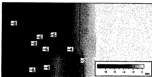
図-3 地表面の鉛直変位分布
