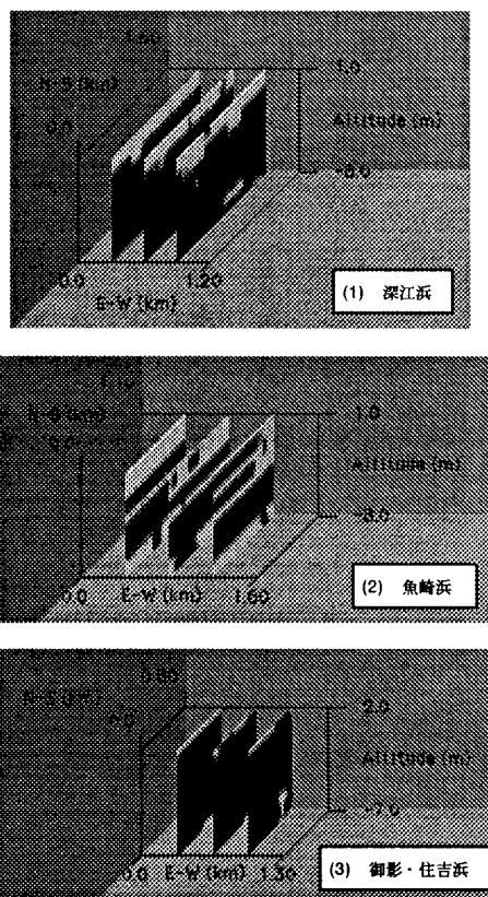
図3 液状化領域の三次元分布
