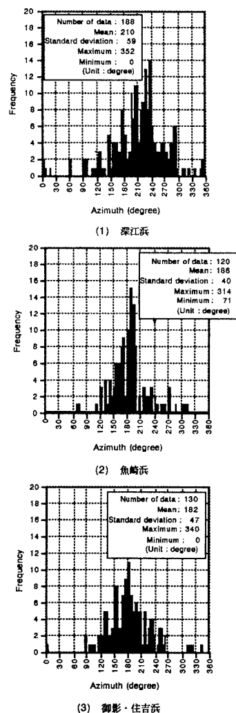
図1 側方流動方位角のヒストグラム
