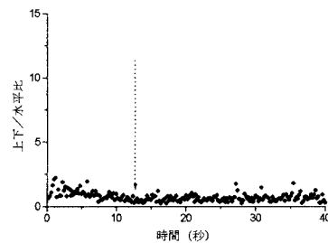
図 5 千早赤阪での上下／水平比
