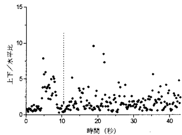
図 4 ポートアイランドでの上下／水平比
