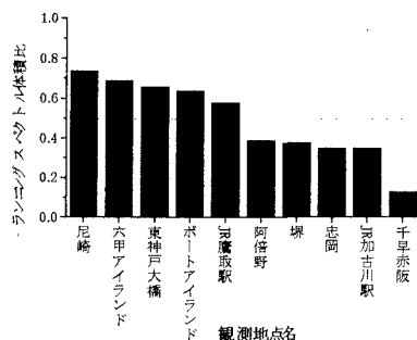
図 3 各観測地点のランニングスペクトル体積比
