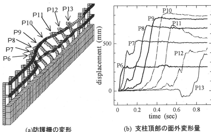
図-3 衝突後の防護柵の変形
