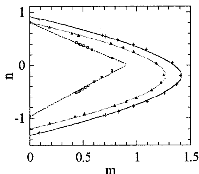
図-4 充填断面の各種強度曲線
