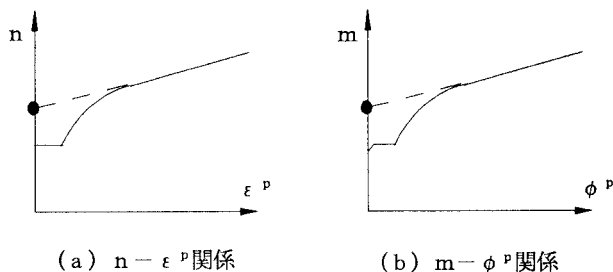
図-3 境界曲線のサンプルポイントの概念図
