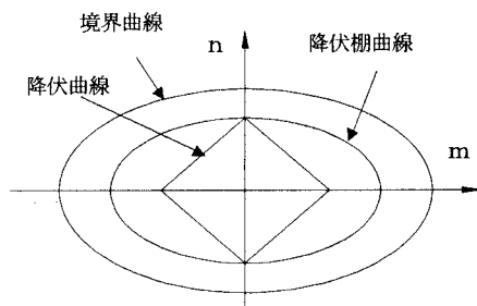
図-5 鋼部材断面の各種強度曲線
