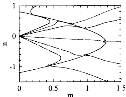
図-2 降伏棚曲線の計算
