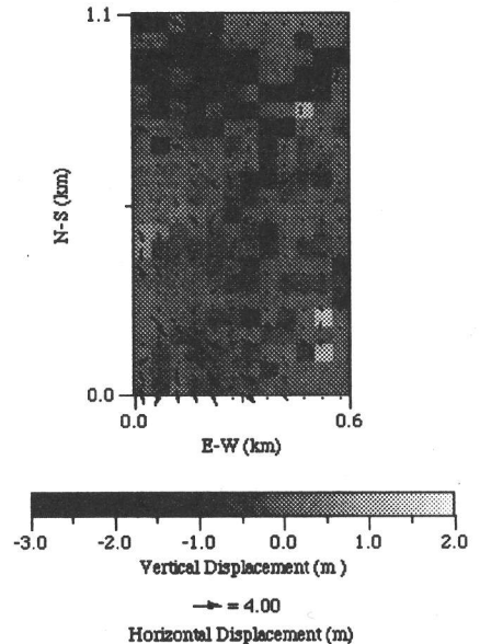
図1 地盤変位
