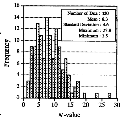
図3 N 値の分布特性
