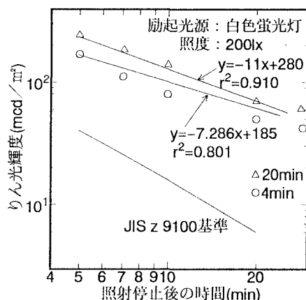
図-1 照射停止後の時間とりん光輝度の関係
