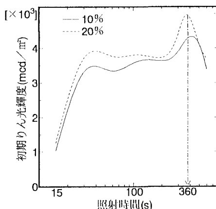
図-3 照射時間とりん光輝度の関係
