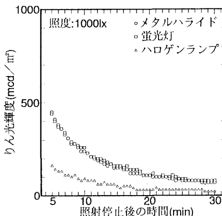
図-4 光源の種類とりん光輝度の関係
