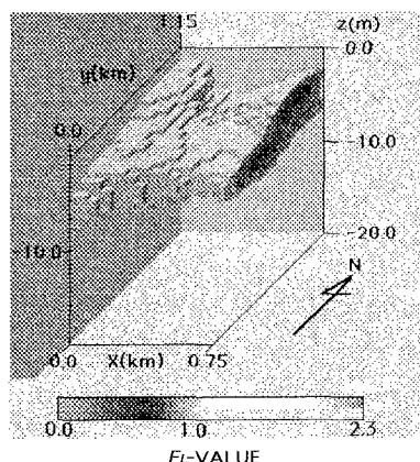
図2 液状化領域の空間分布
