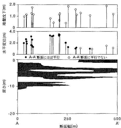
図3 液状化領域と永久変位 (A-A'断面)
