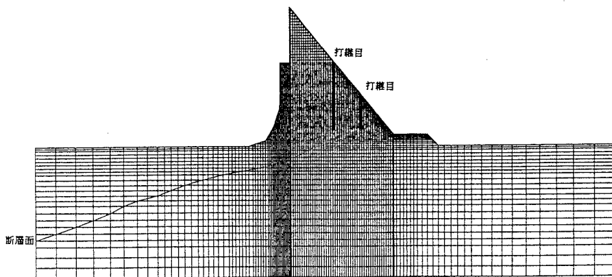
図1 メッシュ図
