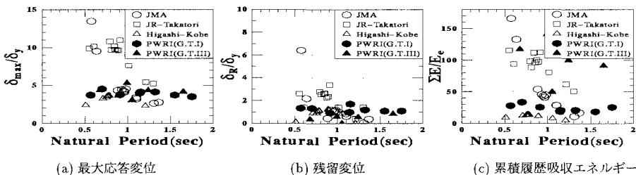
Fig. 2 最大応答変位、残留変位および累積履歴吸収エネルギー
