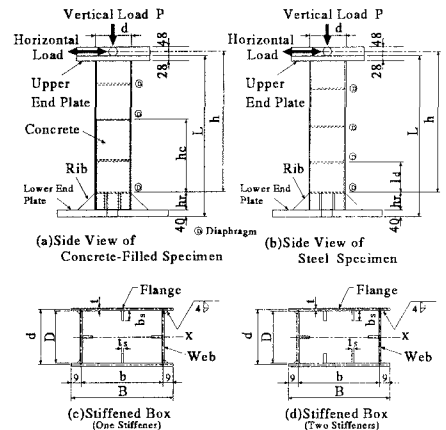
Fig. 1 実験供試体
