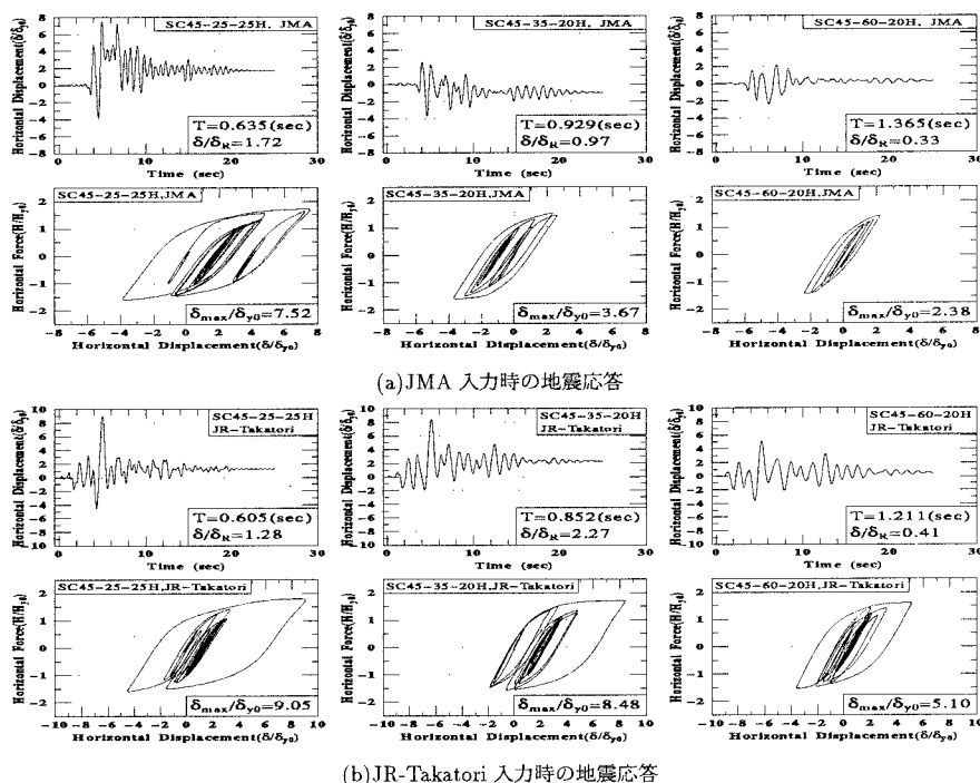
Fig. 3 コンクリート部分充填柱の時刻歴応答変位波形および復元力履歴ループ
