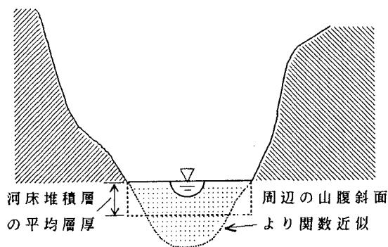
図-3 河谷の断面形状および堆積層厚の推定方法
