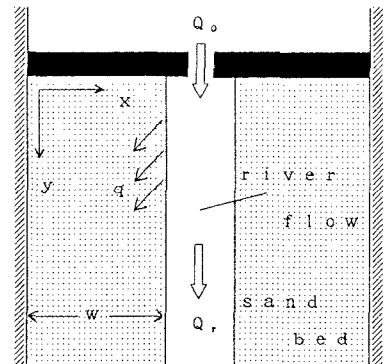
(1) 図-1 理論解析における河川形態
