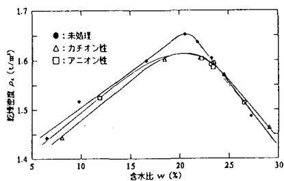
図-1 イオン性界面活性剤処理土の締固め曲線
