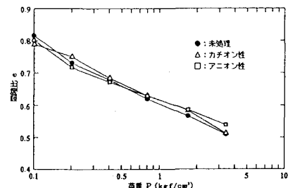
図-3 イオン性界面活性剤処理土のe-log p関係
