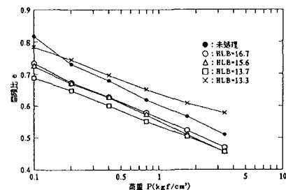
図-4 非イオン性界面活性剤処理土のe-log p関係
