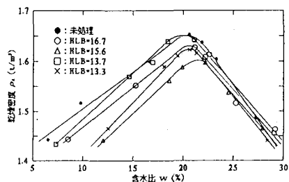
図-2 非イオン性界面活性剤処理土の締固め曲線
