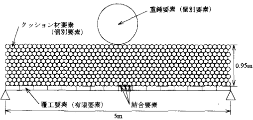
図-1 解析に用いた要素配列
