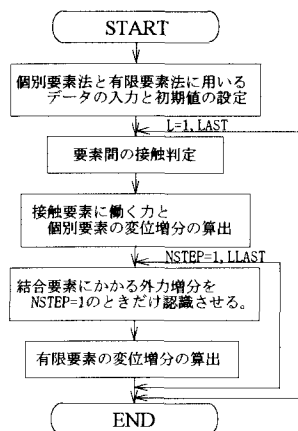
図-2 解析のフローチャート
