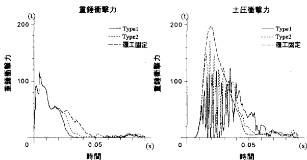
図-3 重錘衝撃力および覆工にかかる土圧衝撃力の変化
