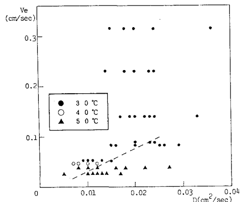
図-3 熱拡散係数 D の同定値と流速 v_0 との関係
