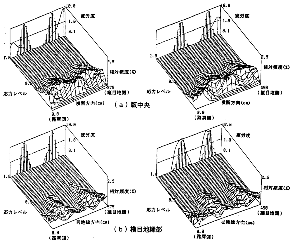
図1 車輪走行位置と疲労度の関係(車線幅:3.5m)
