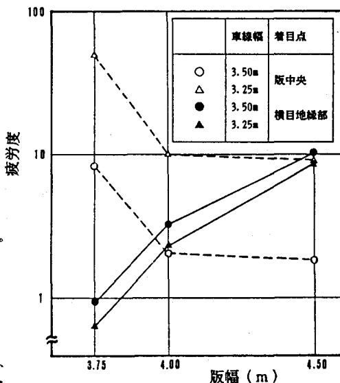
図2 版幅、車線幅および疲労度の関係
