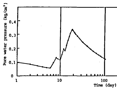
図-4 間隙水圧-時間関係
