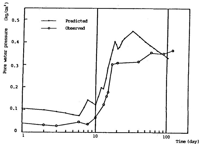
図-3 間隙水圧-時間関係 (要素 29)
