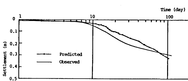
図-2 沈下-時間関係 (盛土中央)
