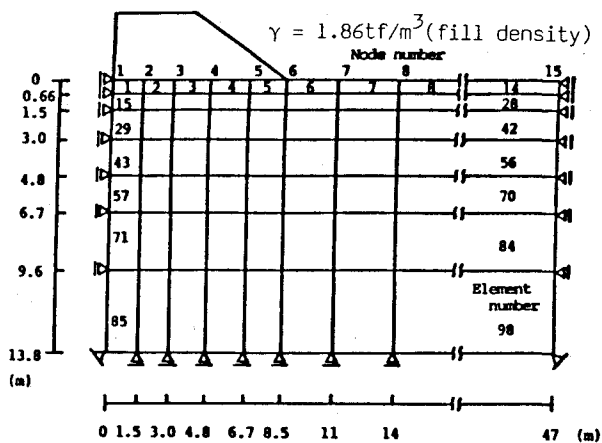
図-1 有限要素メッシュ
