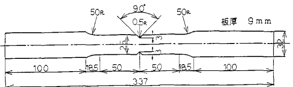
図-1 試験片の形状と寸法
