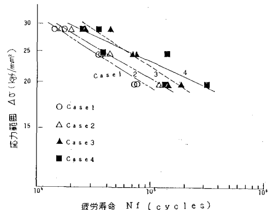
図-2 疲労試験結果
