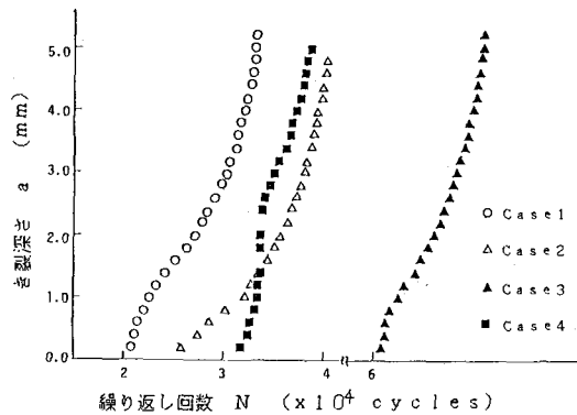
図-4 き裂進展曲線 ( \Delta\sigma = 24.5 \text{ kgf/mm}^2 )
