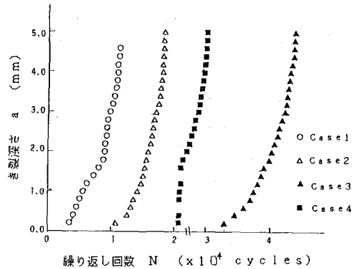
図-3 き裂進展曲線 ( \Delta\sigma = 29 \text{ kgf/mm}^2 )
