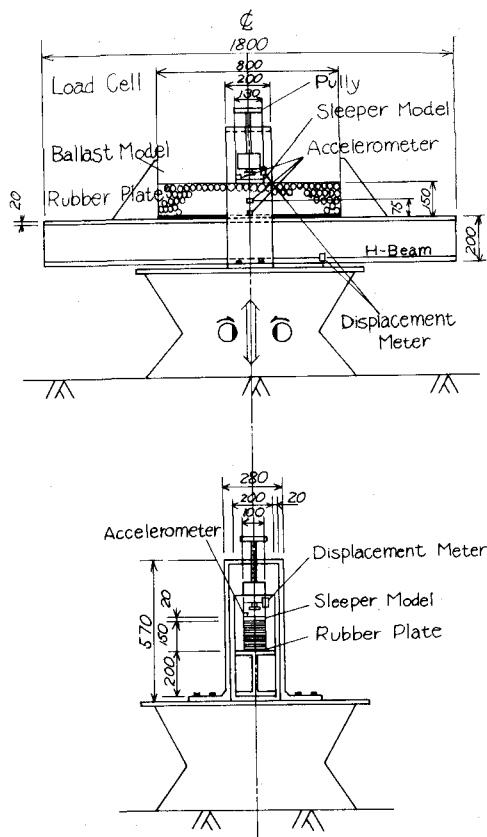
図-1 加振実験装置概略(縦断面, 横断面)
