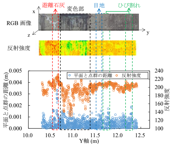
Fig.4 反射強度と幾何学指標による損傷評価
