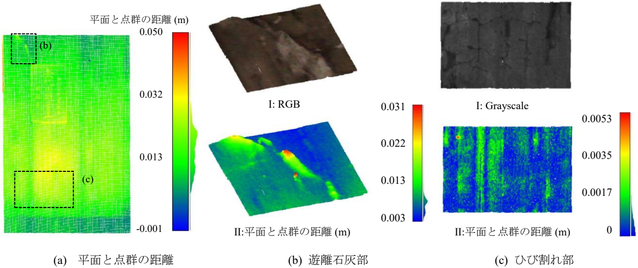
Fig.3 平面と点群の距離による損傷検出
