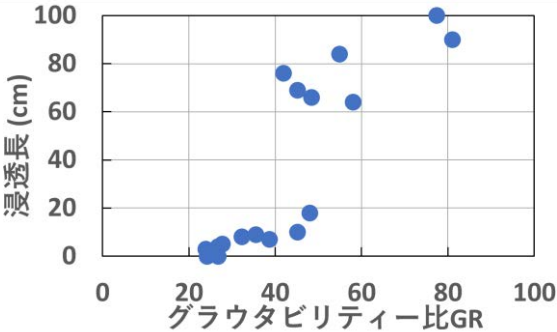
図 3.3 グラウタビリティー比と浸透長関係
