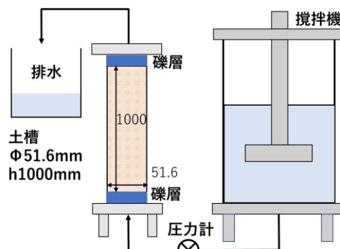
図 2.1 注入装置概要図
