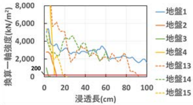
図 3.2 針貫入試験結果
