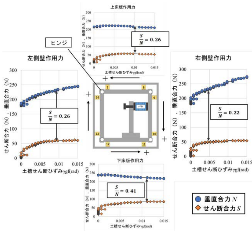
図-4 ヒンジ型函体模型の外観と各面に作用する力の関係図
