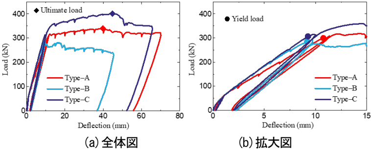
図ー2 荷重－スパン中央変位関係
