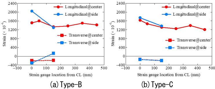
図ー3 引張側 I 形鋼ウェブのひずみ分布
