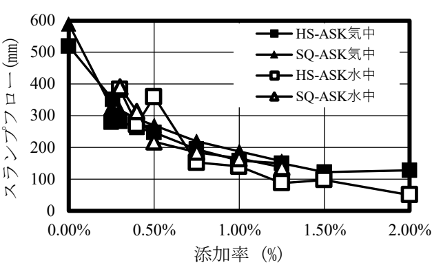
図-3 ASK スランプフロー
