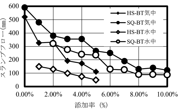
図-2 BT スランプフロー
