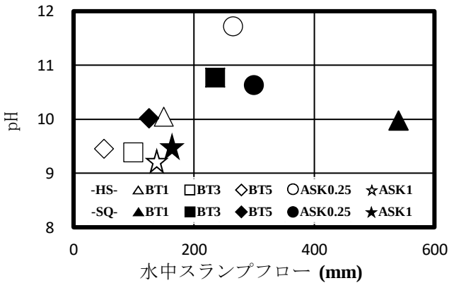
図-4 水中スランプフローと水槽水 pH
