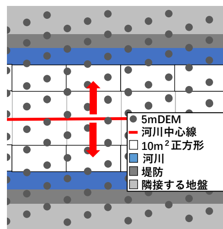
図-2 河道断面特性設定手法
