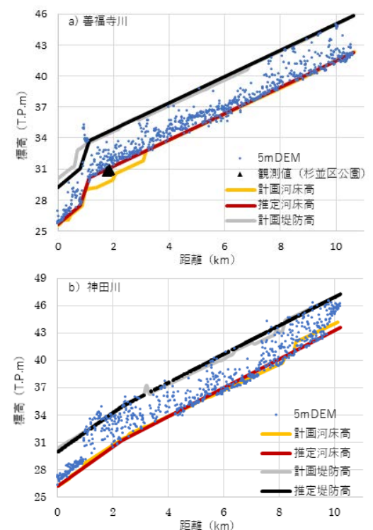
図-5 河床高・堤防高の推定
