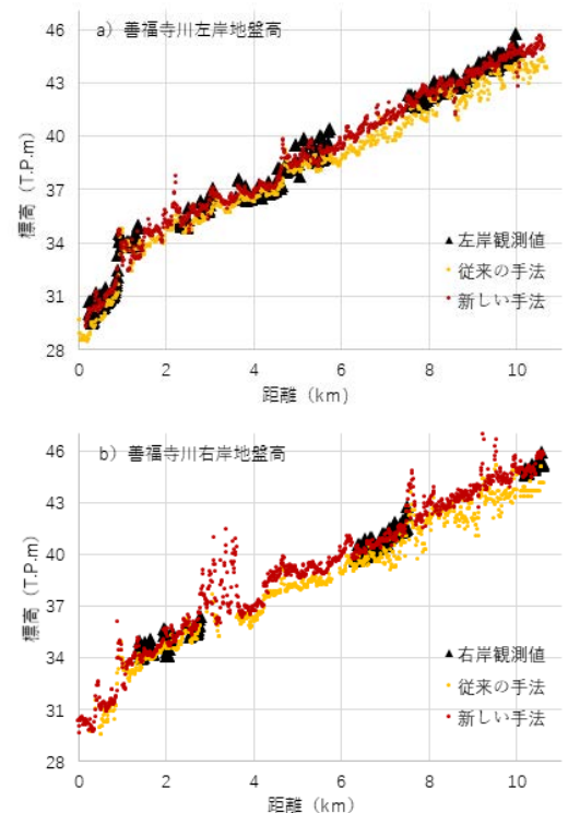
図-4 善福寺川沿い地物の地盤高推定
