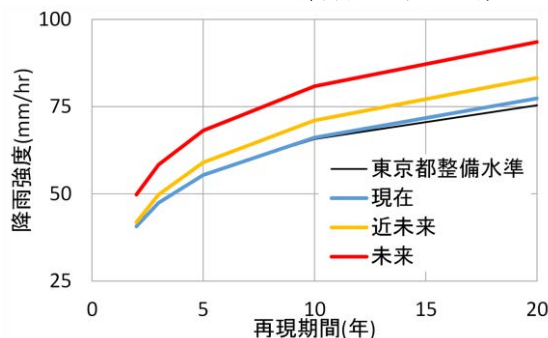
圖-2 確率降雨強度曲線
