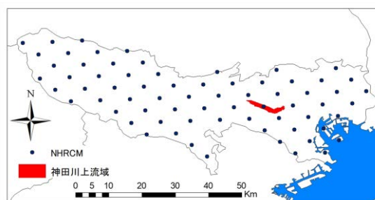
図-1 NHRCM 5Km 解析格子中心座標
