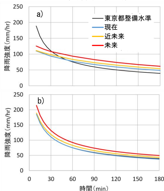
図-3 年超過確率 1/20 の降雨強度曲線
