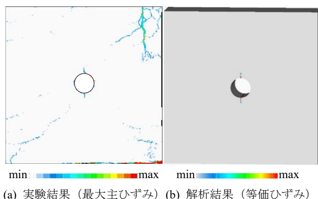
図-2 ひび割れ発生初期のひび割れの比較
