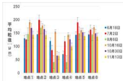
図-3 土壌粒径
