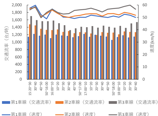
図-1 10 分間交通流率と平均速度
