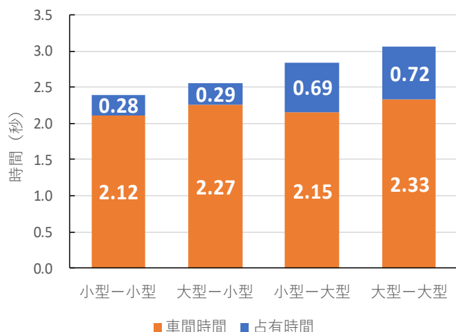
図-2 車間時間と占有時間
