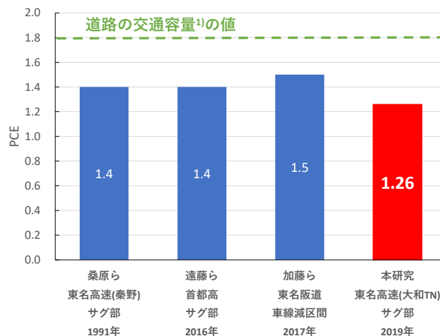
図-3 既往研究との PCE の値の比較
