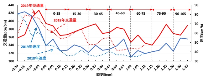
図-1 交通量と速度変化図
