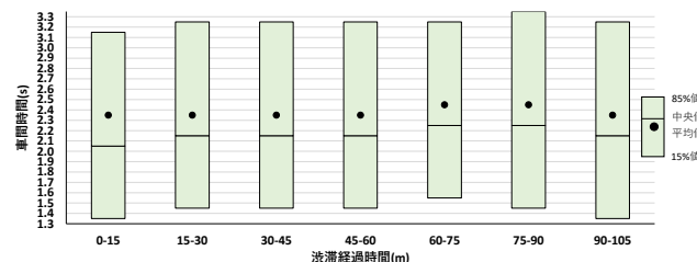
図-3 2019年車間時間の代表値
