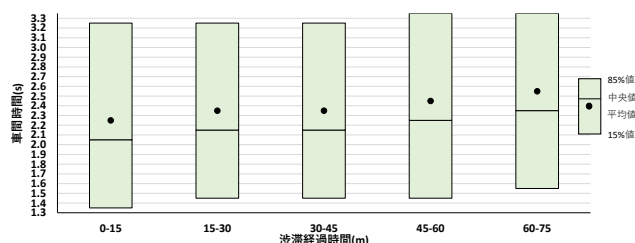
図-2 2018年車間時間の代表値
