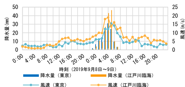
図-4 2つのアメダス観測点における気象データ (2019年9月8日～9日)
