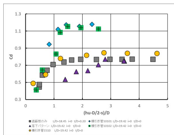
図2 下流側横引き管流入口での流量係数
