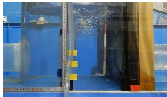
写真1 マンホール内の流況( d=10\text{cm}, \text{case5} )
