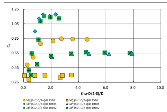
図3 上, 下流側の横引き管流入口での流量係数
