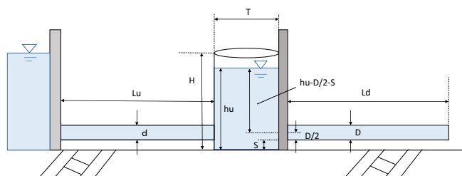
図1 実験模型概略図
