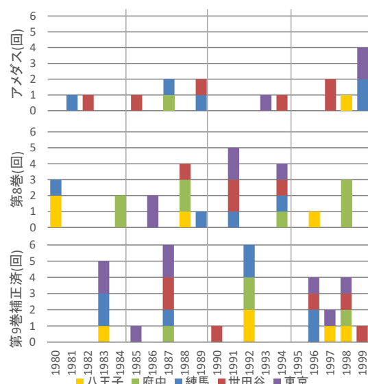
図-2 1時間降水量50mm以上の発生回数(現在気候)
