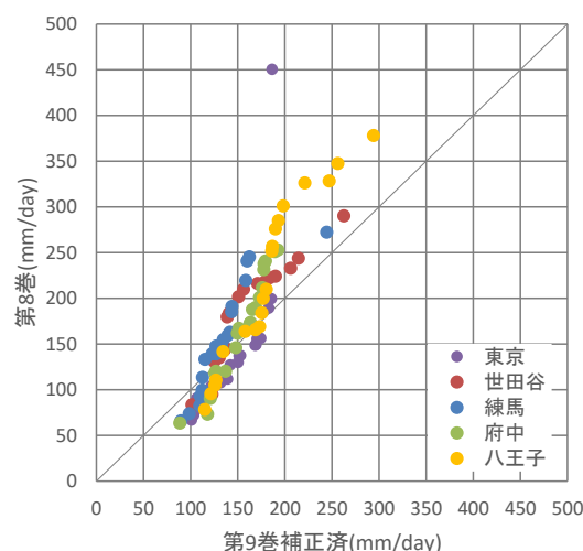
図-3 将来気候の年最大日降水量
