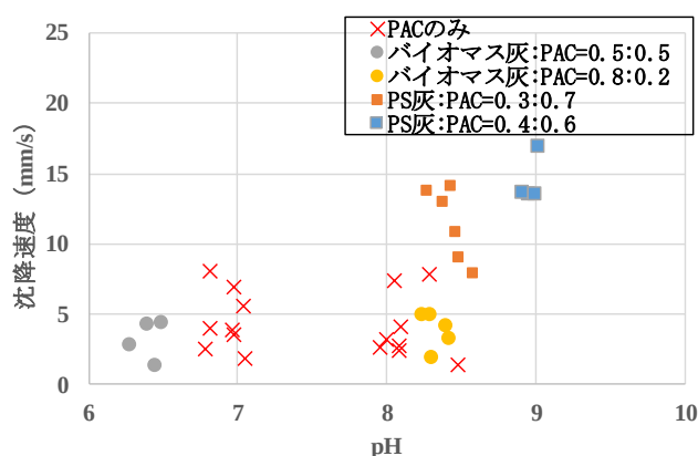
図 2 各サンプルの沈降速度
