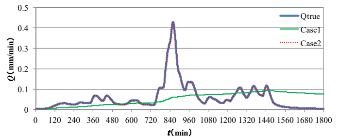
図-2 同定値によるハイドログラフ
