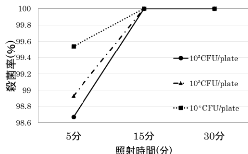
図-3 大腸菌の殺菌率の経時変化
