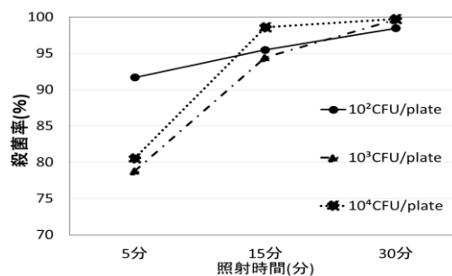
図-5 酵母の殺菌率の経時変化
