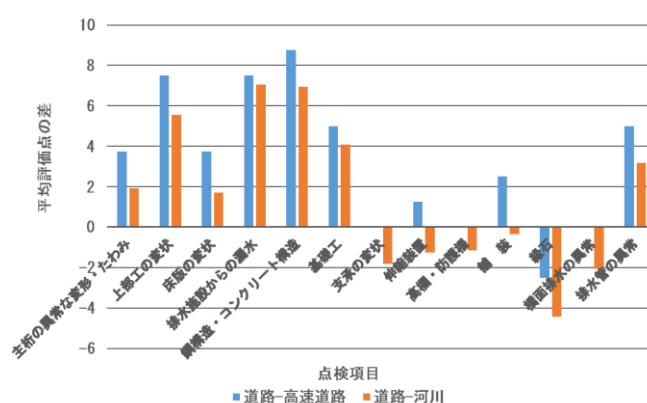
図5 橋下を通るものの別評価点平均の差
