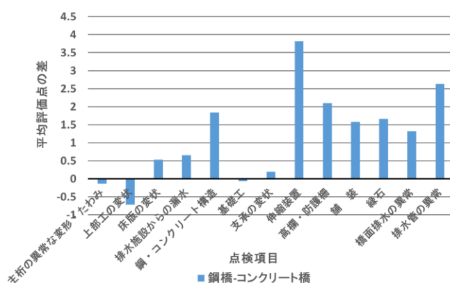
図4 橋梁種類別項目別評価点平均の差
