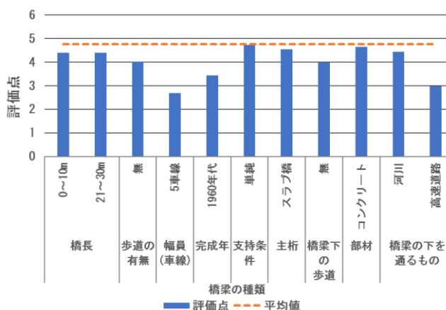
図2 平均評価点以下の橋梁種類別評価点
