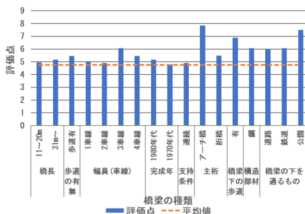
図1 平均評価点以上の橋梁種類別評価点
