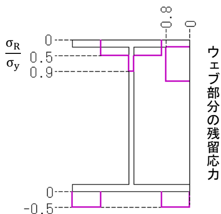
図-2 モデルに取り入れた残留応力分布図 2)
