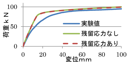
図-4 強軸補強後の荷重-変位グラフ
