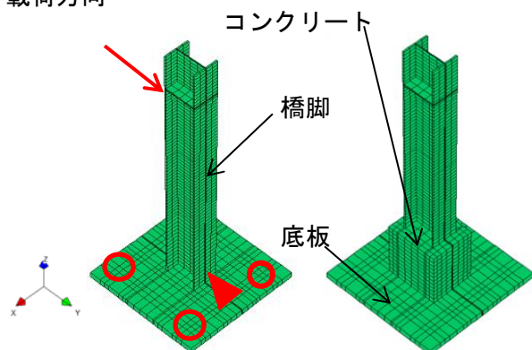
図-1 FINAL 解析モデル 補強前と補強後
