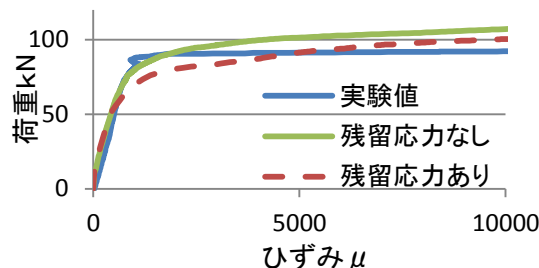
図-5 荷重-ひずみグラフ
