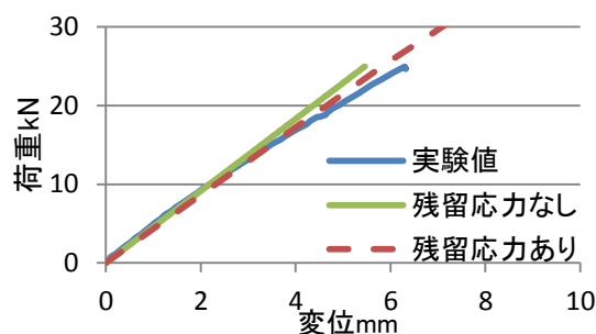
図-3 強軸補強前の荷重-変位グラフ
