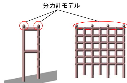
図-5 解析用堰堤モデル
