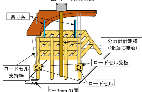
図-2 堰堤モデルと荷重計測要領
