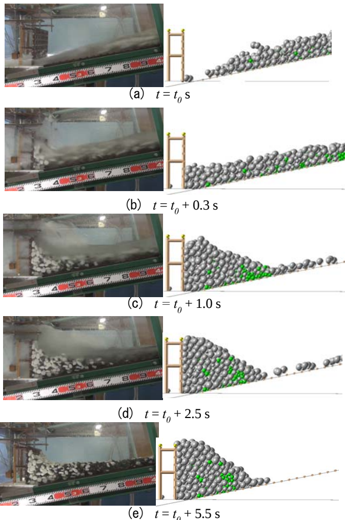
図-4 捕捉堆積過程 (左:実験, 右:解析)
