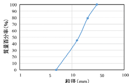
図-3 粒径加積曲線
