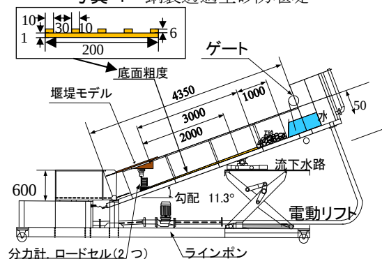
図-1 実験水路
