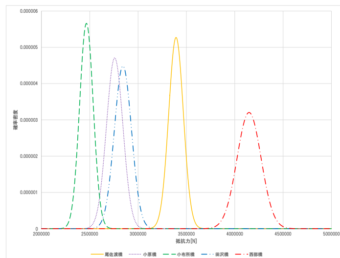
図-2 抵抗力の確率密度関数
