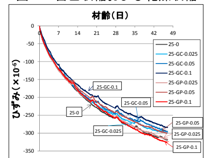
図-4 乾燥収縮 (W/C=25%)
