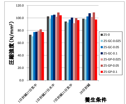
図-2 圧縮強度 (W/C=25%)
