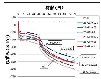
図-3 自己収縮および乾燥収縮
