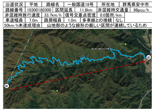
図－7 50km/h 未達成区間の確認
