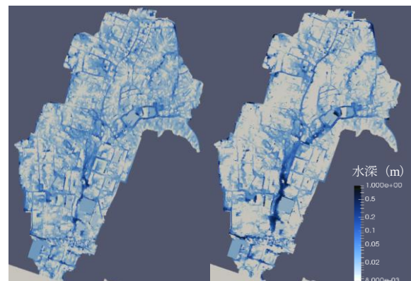
図-5 VTK による浸水深表示 (左:40 分後, 右:60 分後)
