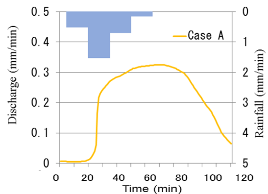
図-4 Kyrkviken 湾への流出量
