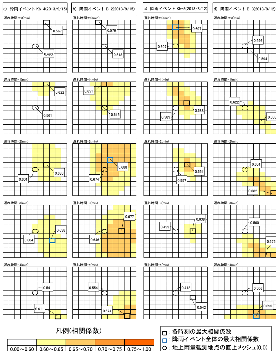
図-5 地上雨量と観測地点周辺メッシュにおけるXバンドMPレーダ雨量の相関係数の時空間分布
