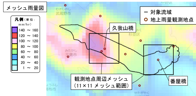
図-7 X バンド MP レーダ雨量状況 (降雨イベント Kb-3 8/12 18:25 時点)
