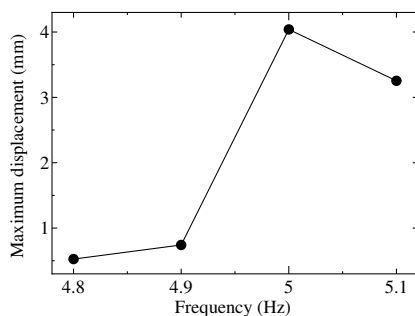
図-3 最大浮上り変位と加振振動数の関係
