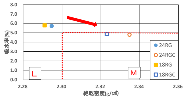
図-1 再生粗骨材の密度・吸水率試験結果
