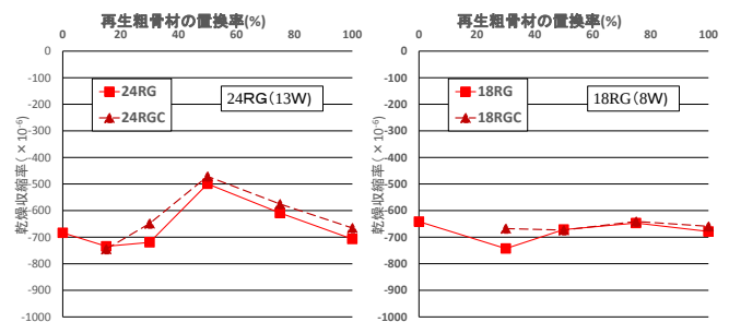
図-3 乾燥収縮率試験結果
