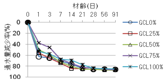
図-9 通水量減少率
