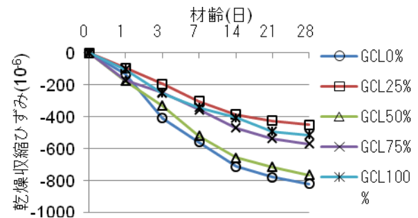
図-7 モルタルの乾燥収縮ひずみの変化
