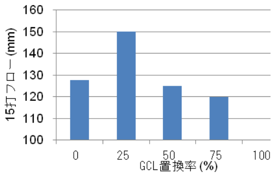
図-3 モルタルの15打フロー
