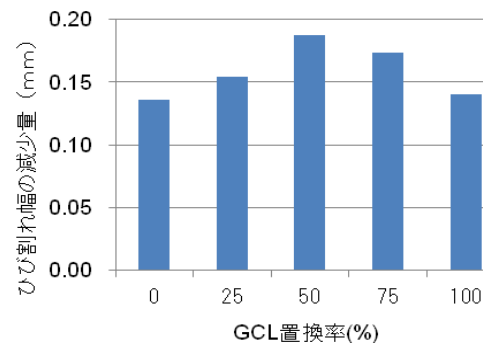
図-10 想定ひび割れ幅の減少量
