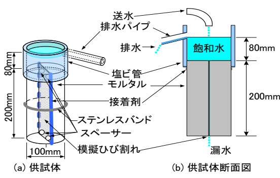
2 通水試験の供試体
