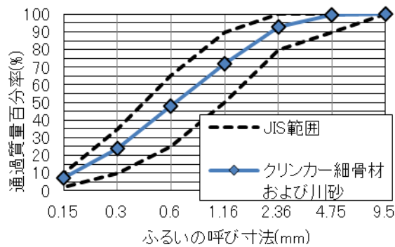
図-1 粒度分布
