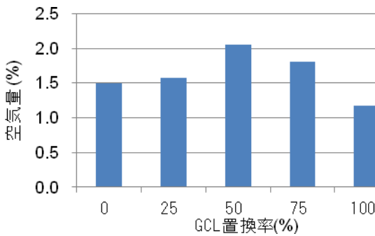
図-4 モルタルの空気量
