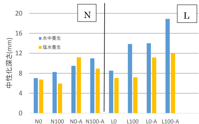
図-3 促進中性化試験
