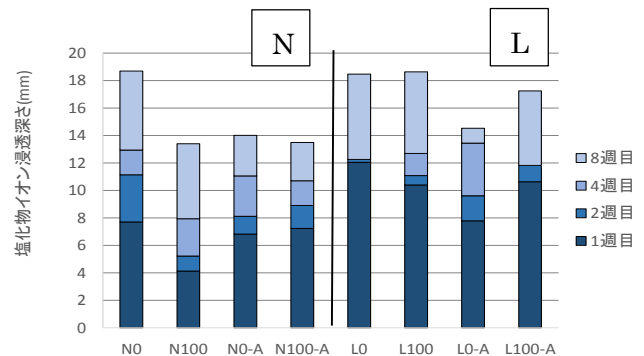
図-2 塩水浸漬試験
