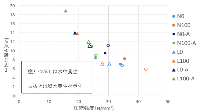
図-4 圧縮強度と中性化深さの関係
