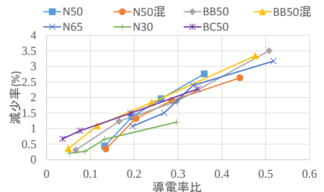
図-5 導電率比と減少率
