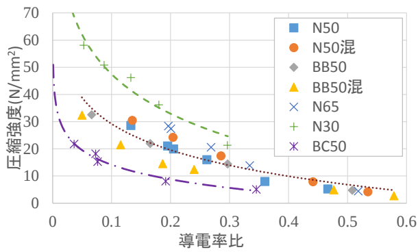
図-1 導電率と圧縮強度
