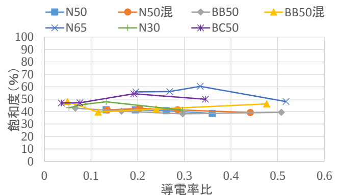
図-4 導電率比と飽和度
