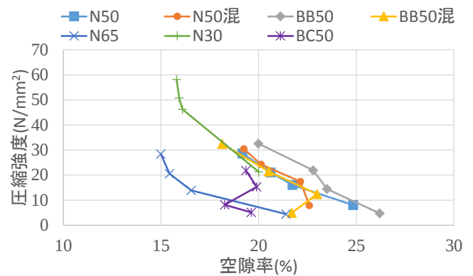
図-2 空隙率と圧縮強度
