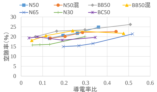
図-3 導電率比と空隙率
